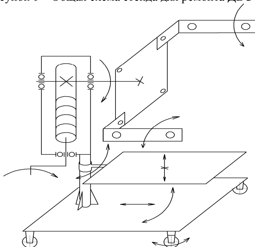
Рисунок 2 – Функциональная (кинематическая) схема стенда для ремонта ДВС
